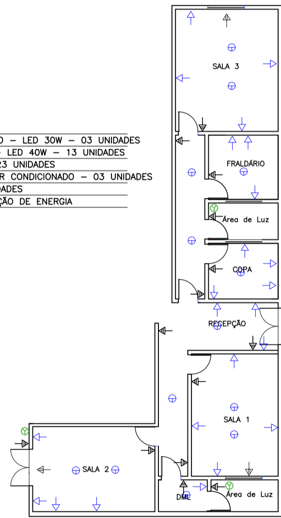
PLANTA BAIXA - LOCAÇÃO DOS PONTOS ELÉTRICOS
