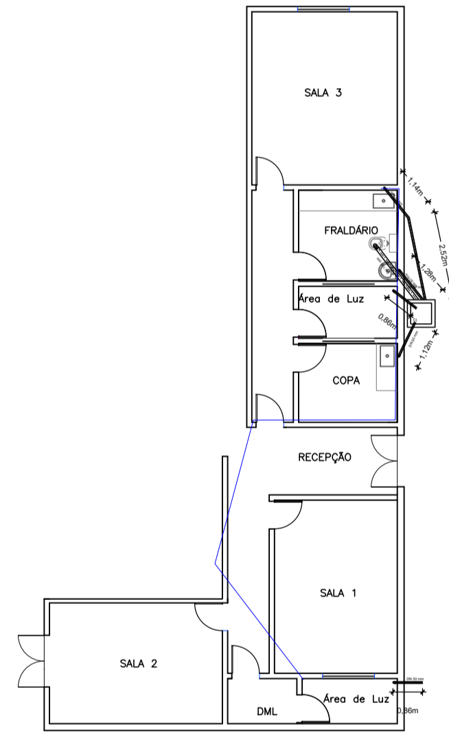
PLANTA BAIXA - HIDRÁULICA
