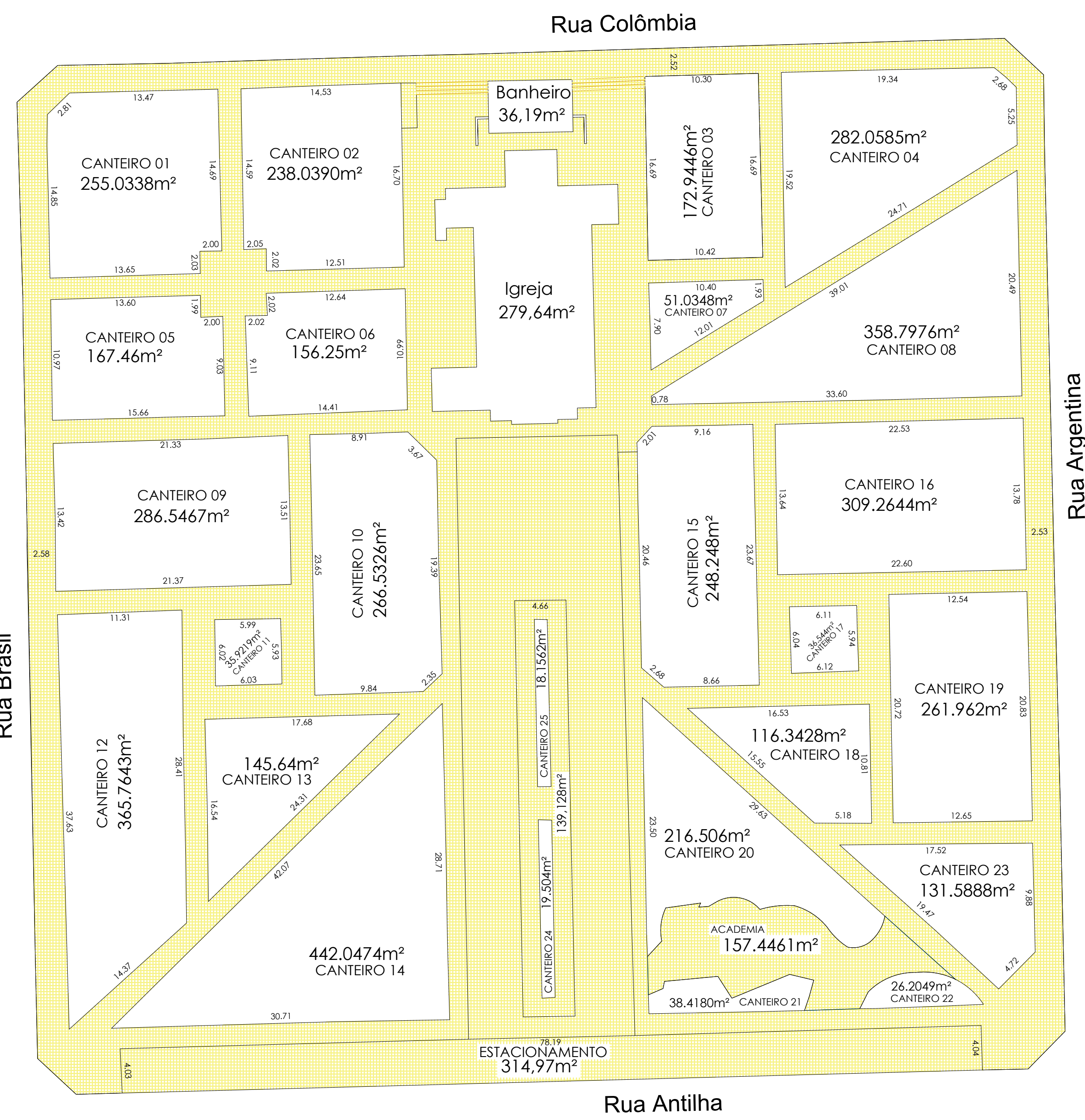
PLANTA BAIXA - DEMOLIÇÃO DO PISO 1:300
