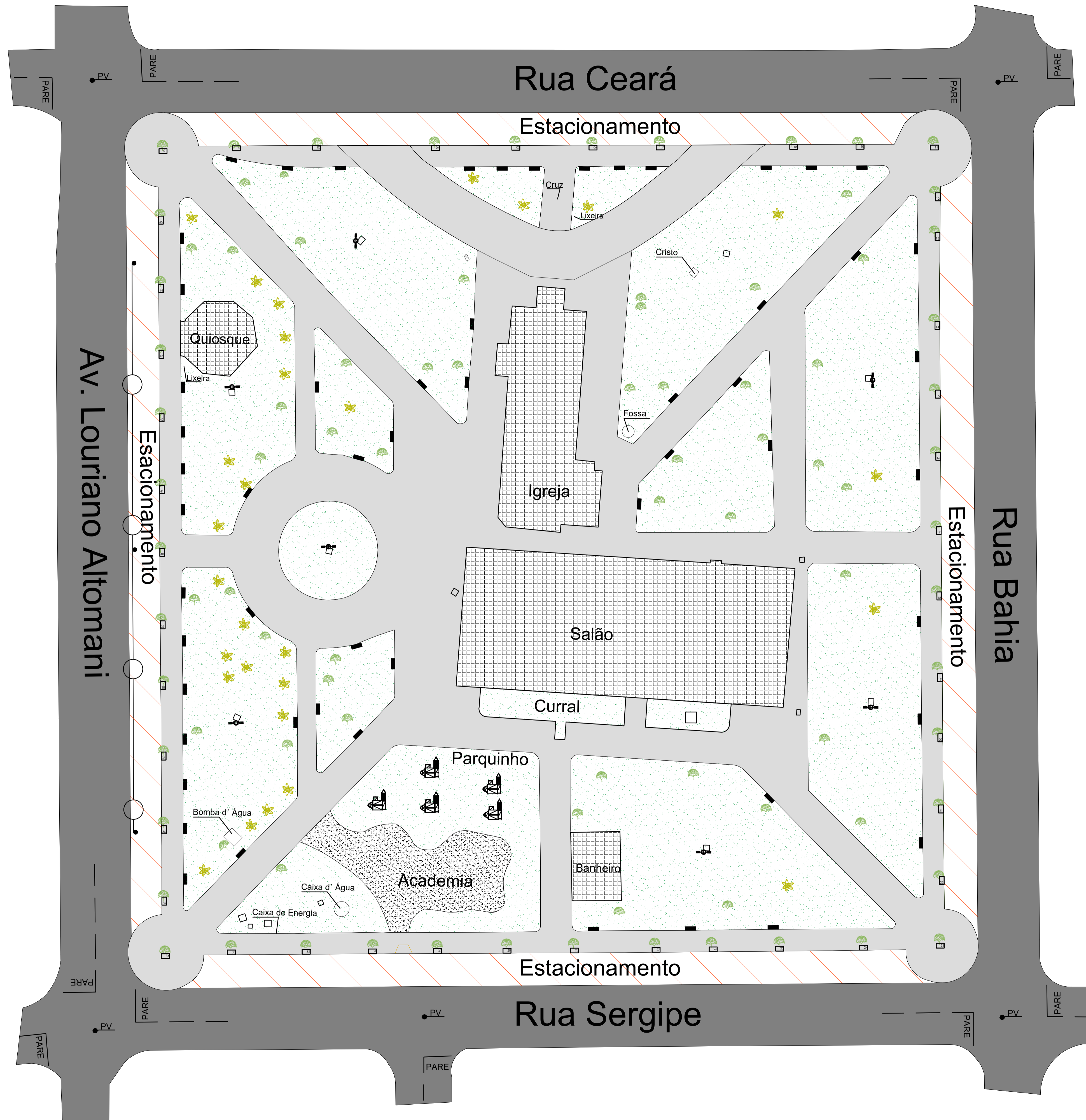
PLANTA BAIXA - SITUAÇÃO ATUAL 1:300
